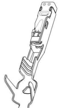
Fig. / Abb. 8: Wire and Insulation Crimp Dimensions / Draht- und Iso-Crimpmaße MCON 1.2 LL SWS
