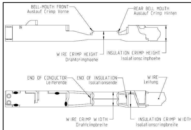
Fig. / Abb. 2: Contact with Wire Insulation Crimp / Kontakt mit Crimp für Leitungsisolierung
